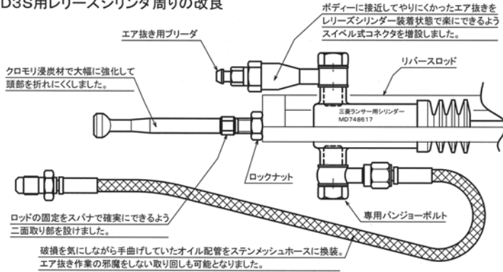
FD3S用レリーズシリンダ周りの改良
